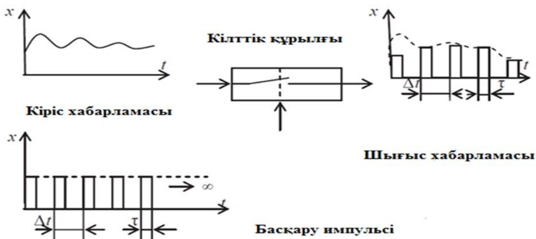
Сурет 3 - Кілттің көмегімен уақыт бойынша үздіксіз хабарларды дискретизациялау
