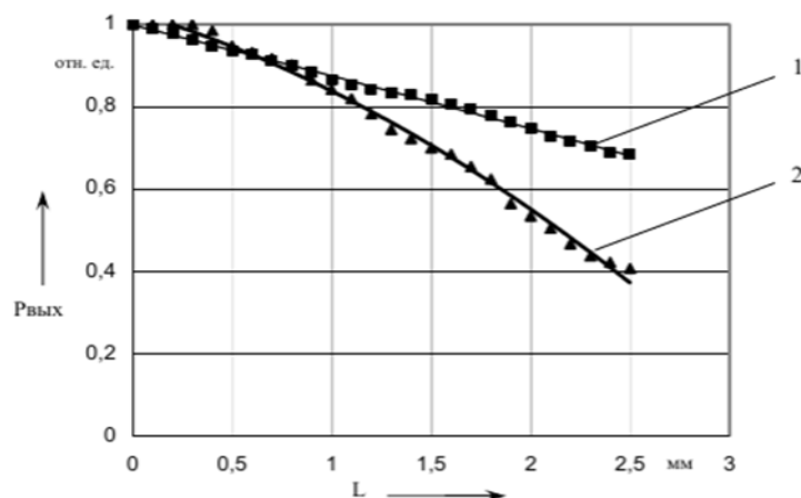
Сурет 4 – Тензодатчиктің шығыс сигналының созылу-қысу деформациясына тәуелділігі: 1-бір бұрылыс сенсоры үшін; 2-11 бұрылыс сенсоры үшін
