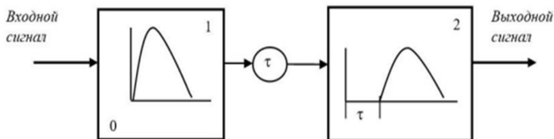
Сурет 1- Артта қалған басқару жүйесінің қарапайым түрі
