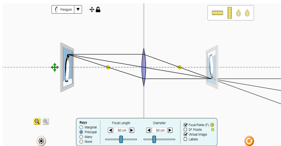
Рисунок 1- Геометрическая оптика
