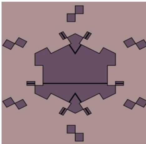
Сурет 2 - Пенрозудың мозаикасы
