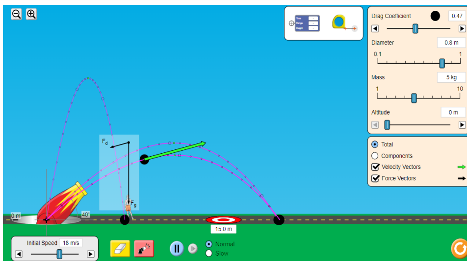
Рисунок 2 - Тело, брошенное под углом к горизонту
