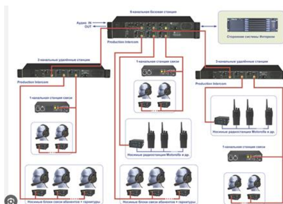
Рисунок 2 – Проводная связь
