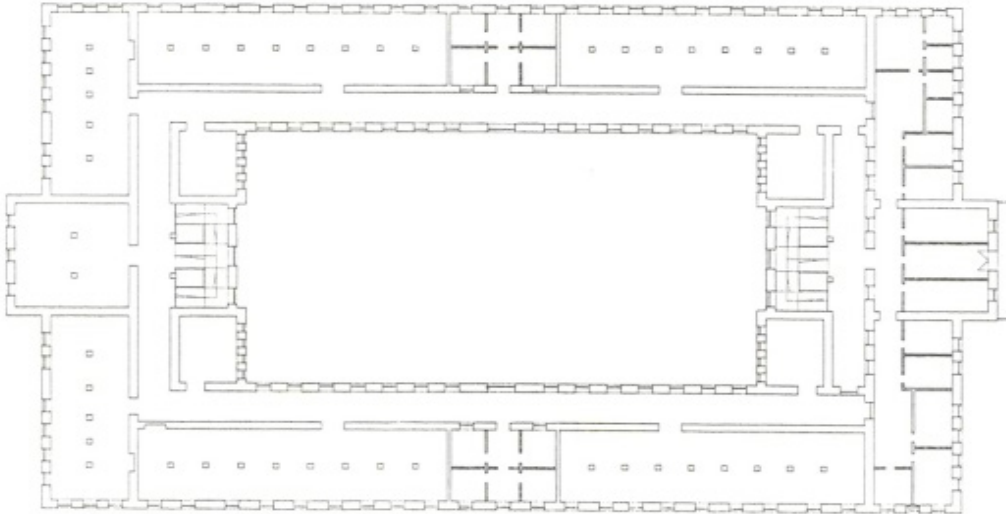
Resim 1 - Manastır askeri idadisi - zemin kat planı (Manastır'da Osmanlı Dönemi Türk Eğitim Yapıları ve Atatürk'ün Okuduğu Askeri İdadi - (Yrd. Doç. Dr. Mehmet Z. İBRAHİMGİL)
